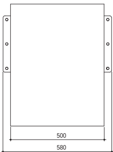
Üstten görünüş
